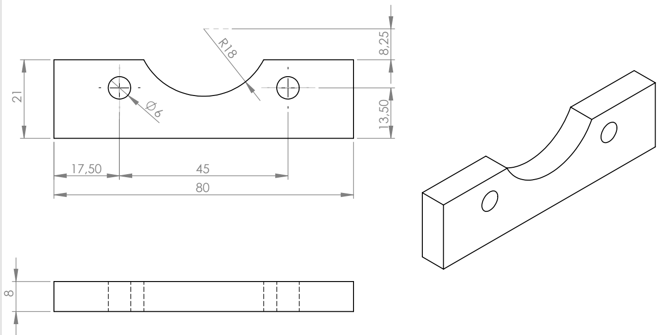
Soporte para os imáns da base Escala 1:1
